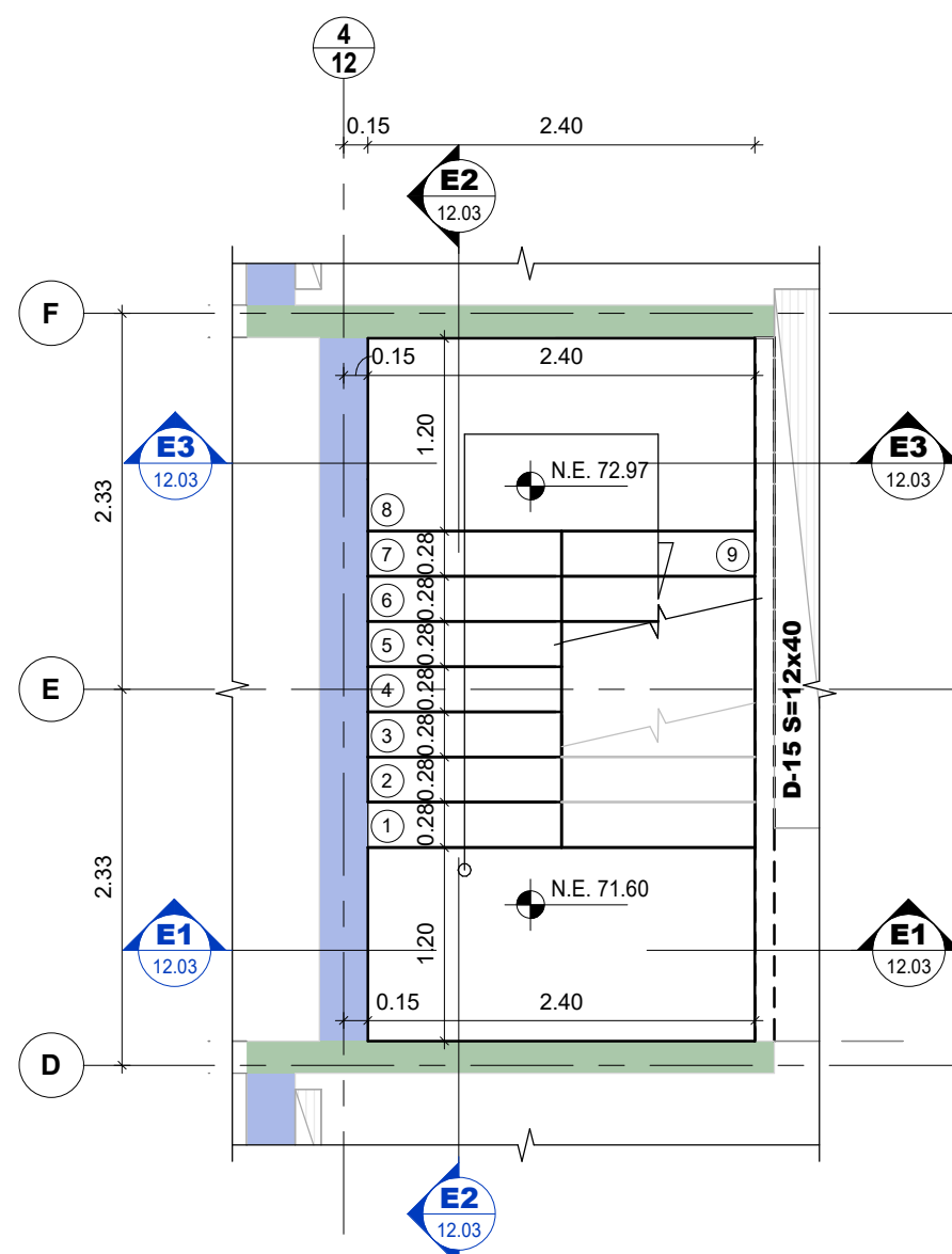
PLANTA ARRANQUE ESCALERA TIPO 1 Y 2 (PISO 28 A CUBIERTA) Escala 1:50
