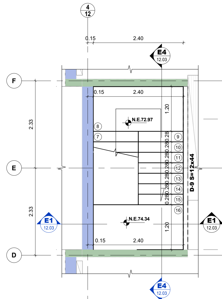
PLANTA LLEGADA ESCALERA TIPO 1 Y 2 (PISO 28 A CUBIERTA) Escala 1:50
