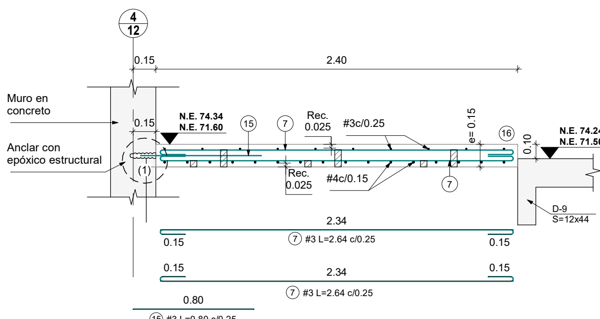
CORTE E-1 Escala 1:25
