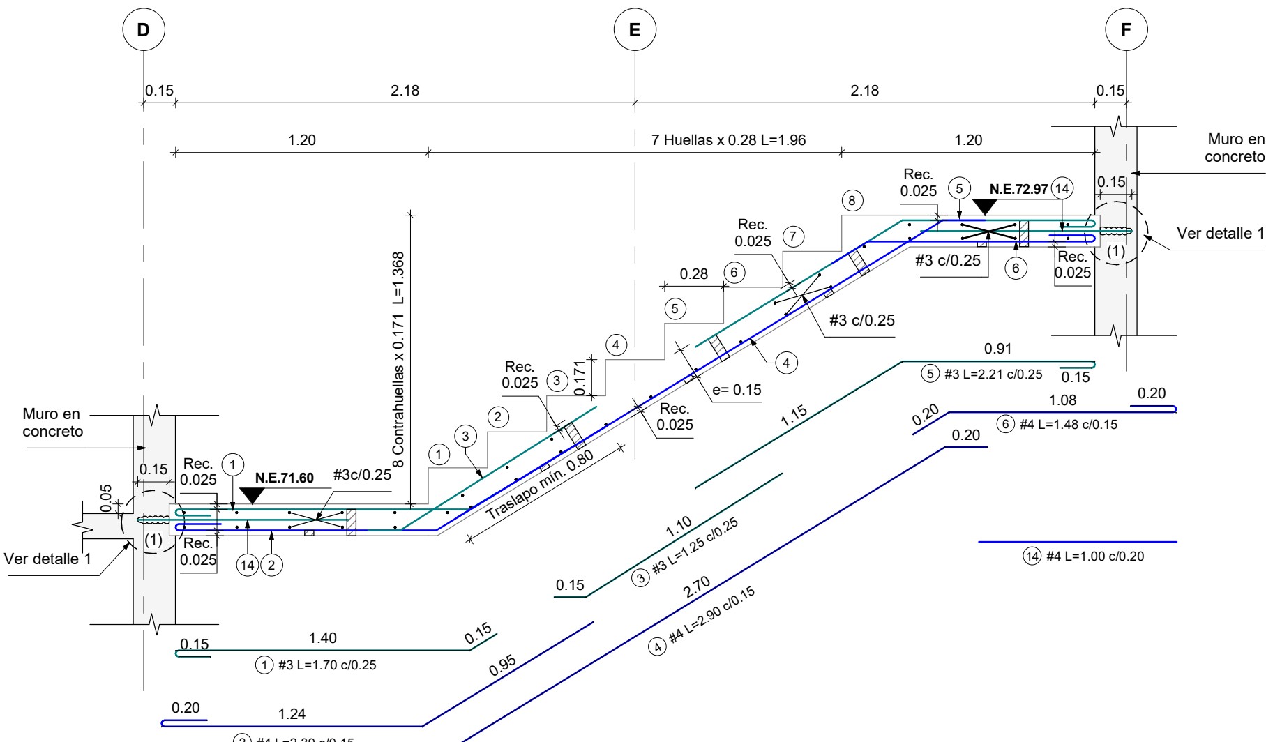
CORTE E-2 Escala 1:25
