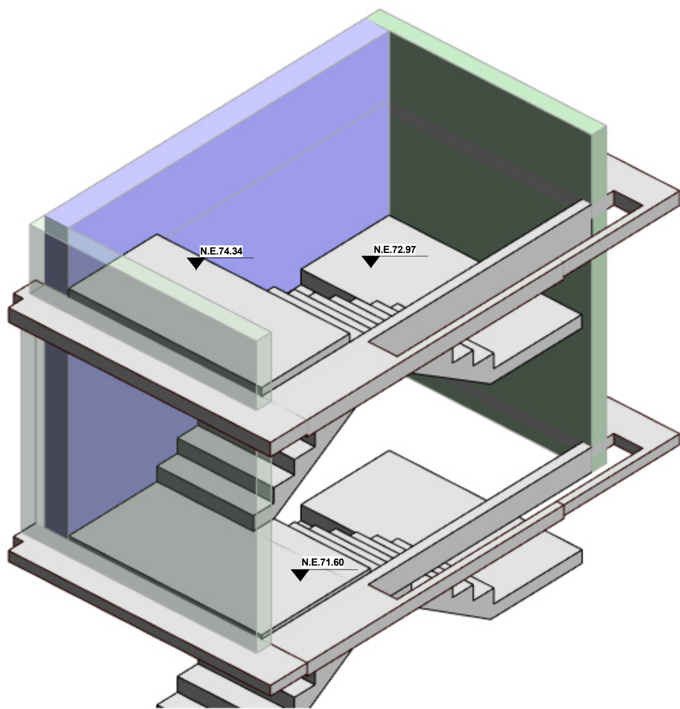
3D ESCALERAS TIPO 1 Y 2 (PISO 28 A CUBIERTA) Sin escala
