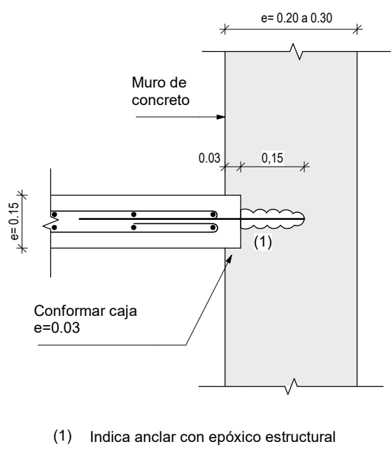
DETALLE 1 Escala 1:10
