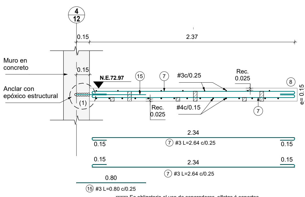
CORTE E-3 Escala 1:25
