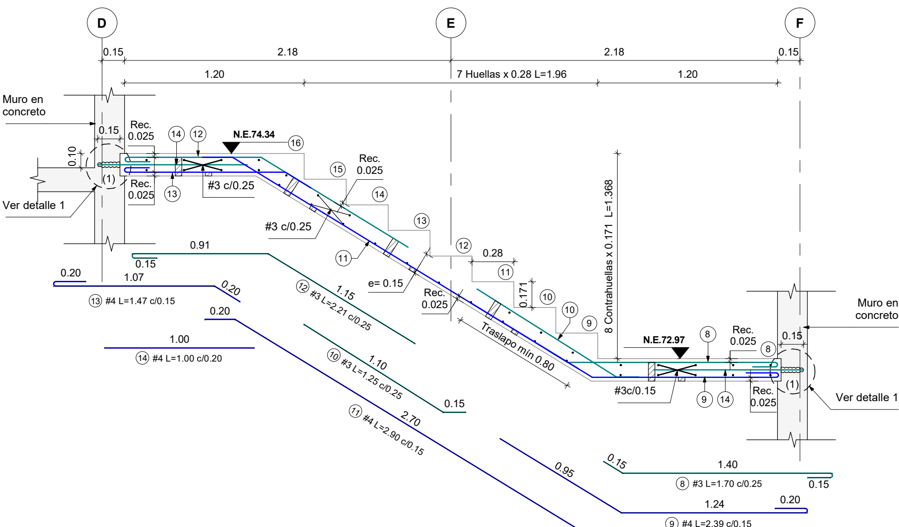
CORTE E-4 Escala 1:25
